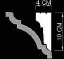
12LK-P (EPS Perdelik)
